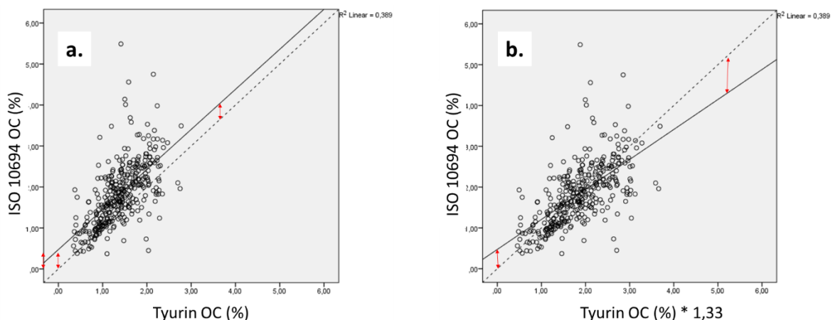
21. ábra. A két módszerrel mért szervesszén-tartalmak összehasonlítása (a.: a Tyurin módszerrel meghatározott OC; b.: a szakirodalom szerint megadott 1,33 konverziós faktorialtal átszámított Tyurin OC)
