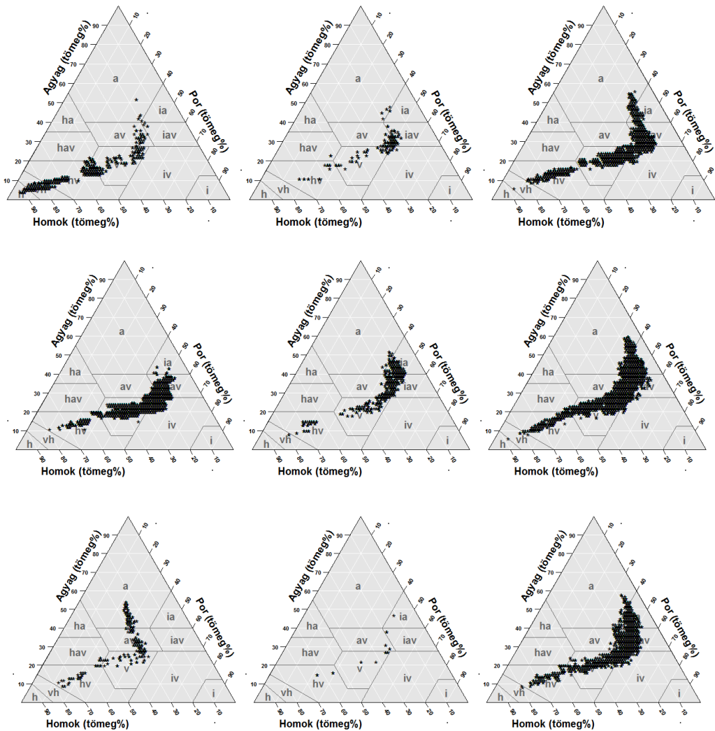
2. ábra. Az AIIR adatbázisban található talaj főtipusok becsült mechanikai összetétele balról jobbra: váztalajok, közethatású talajok, barna erdőtalajok, csernozjom talajok, szikes talajok, réti talajok, láptalajok, mocsári erdőtalajok, öntés- és lejtőhordalék talajok
