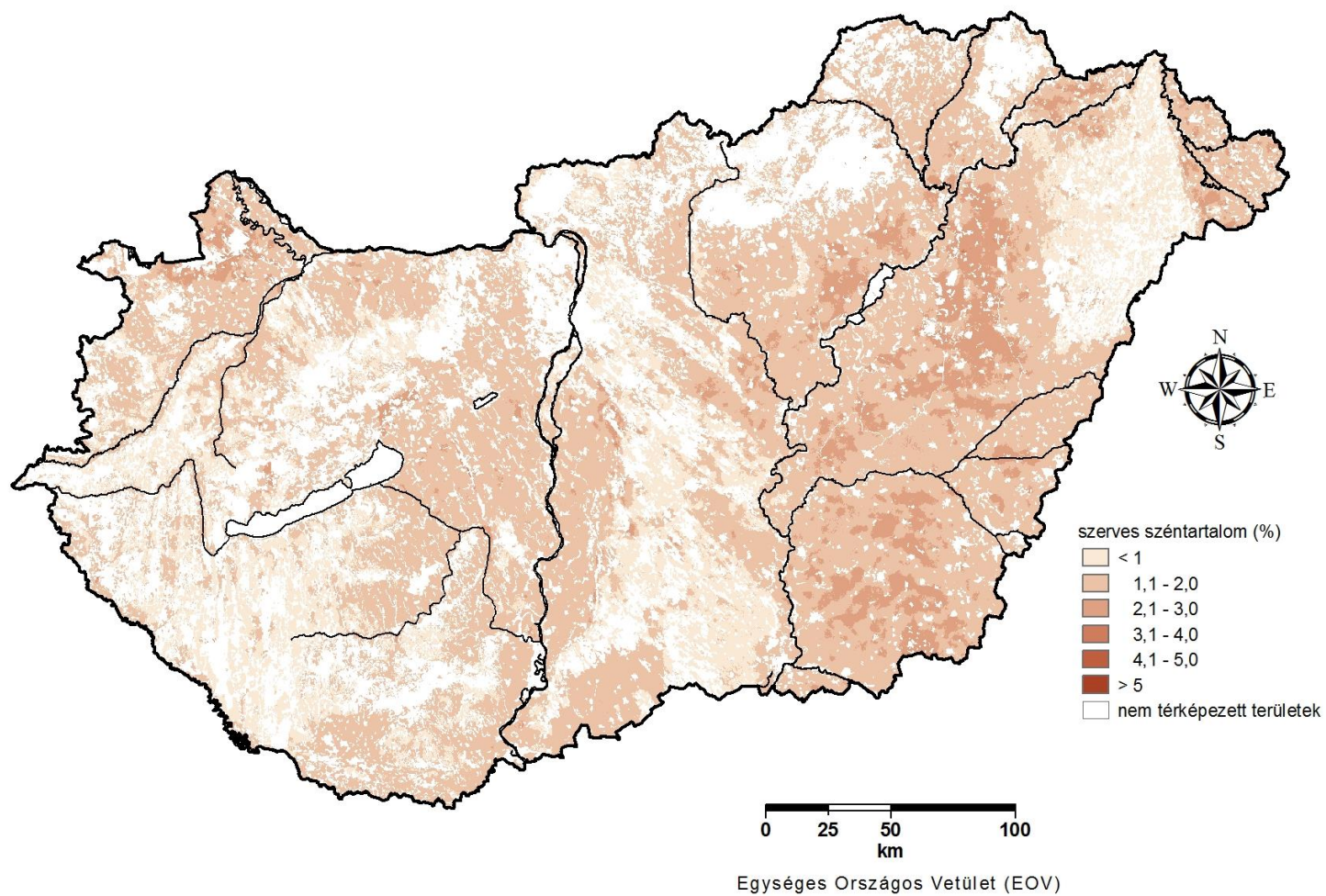
7. ábra. Mezőgazdasági területek feltalajának szerveszén-tartalom térképe (felbontás: 250 m)
