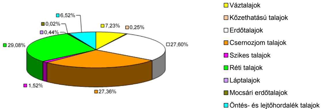
1. ábra. Az AIIR ver3.0 adatbázis talaj főtípusainak területi megoszlása (a mezőgazdasági táblák területe alapján számolva)
